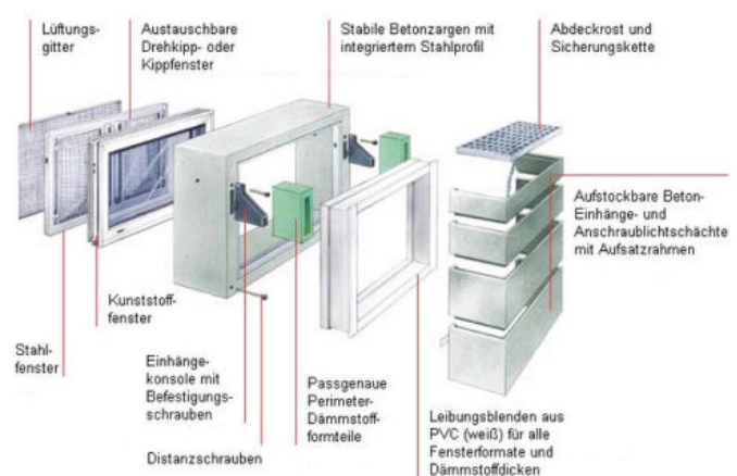
Systemdarstellung UNifix Kombi
