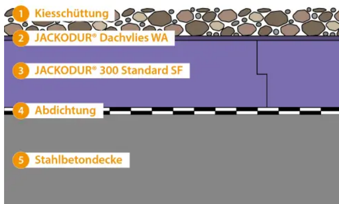
Umkehrdachdämmung bekiest
