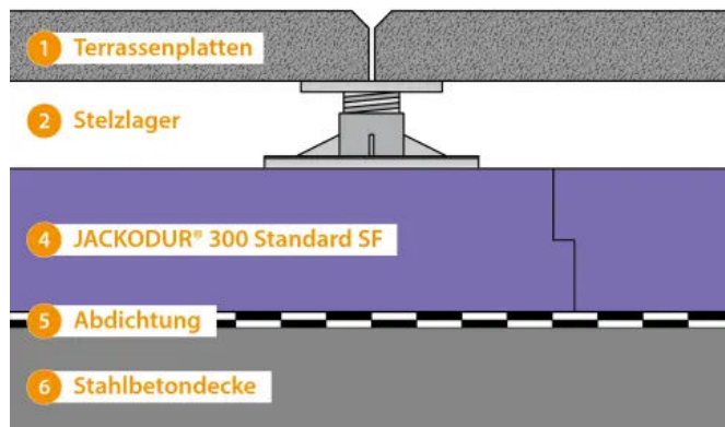
Betonplatten auf Stelzlagern
