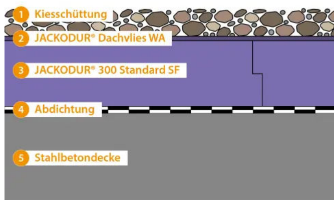
Umkehrdachdämmung bekiest
