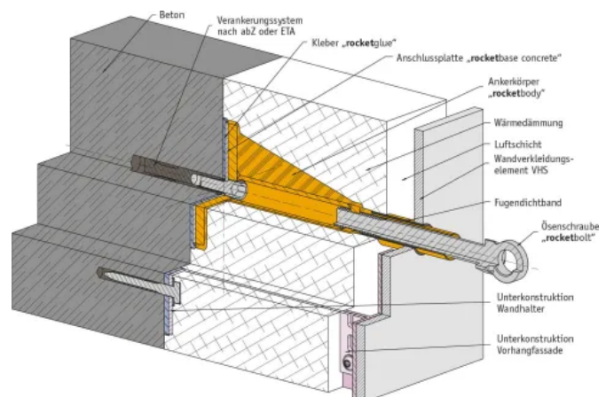
Wandaufbau VHF (abgelengter Ankerkörper)
