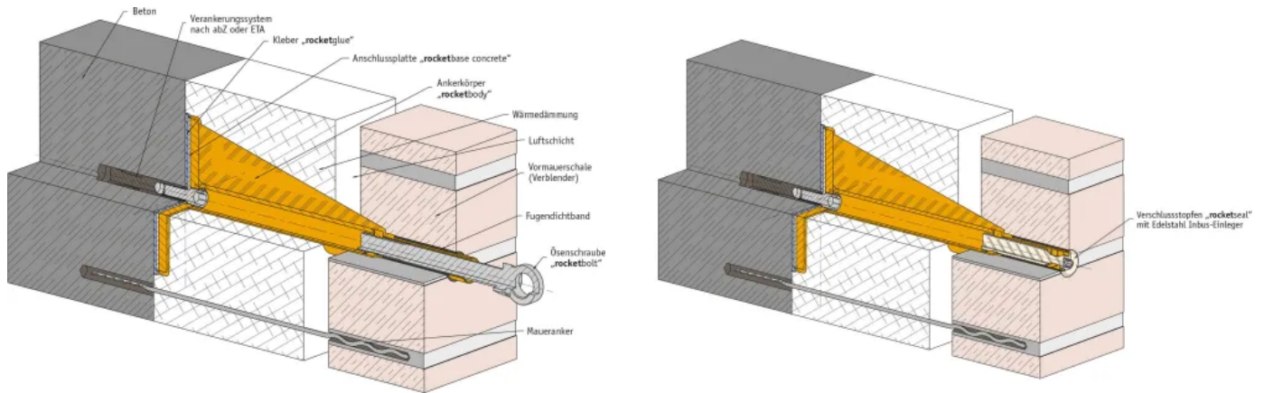
Wandaufbau 2-schaliges Mauerwerk (mit Ankerschraube)
