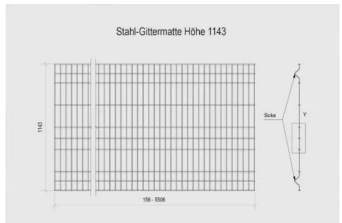
Stahl-Gittermatten 1143 mm
