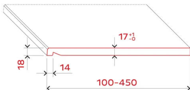
Fensterbanktyp compact
