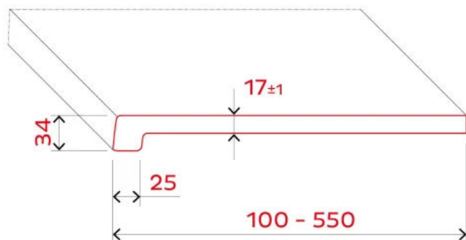
Fensterbanktyp exclusiv
