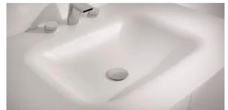
Einzelwaschtisch Bravo L/B von 700/610 mm bis 1400/610 mm Doppelwaschtisch L/B 1220/610 mm und 1520/610 mm
