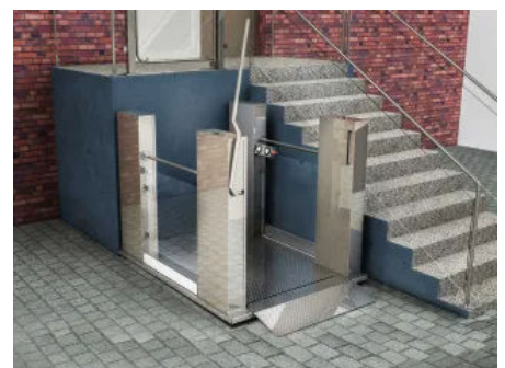
Die robusten Hublifte Vertico Quattro befördern auch schwere Elektro-Rollstühle und E-Mobile bis zu 1.790 mm hoch.
