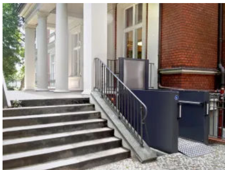
Die integrierte Auffahrrampe des Vertico Intuvo klappt während des Hebens hoch und verhindert ungewolltes Zurückrollen.
