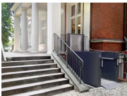
Die integrierte Auffahrrampe des Vertico Intuvo klappt während des Hebens hoch und verhindert ungewolltes Zurückrollen.
