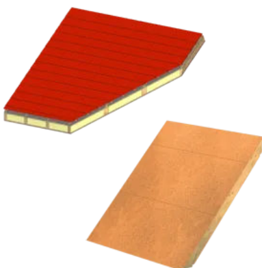
L-SYS Roof Module für das Dach.
