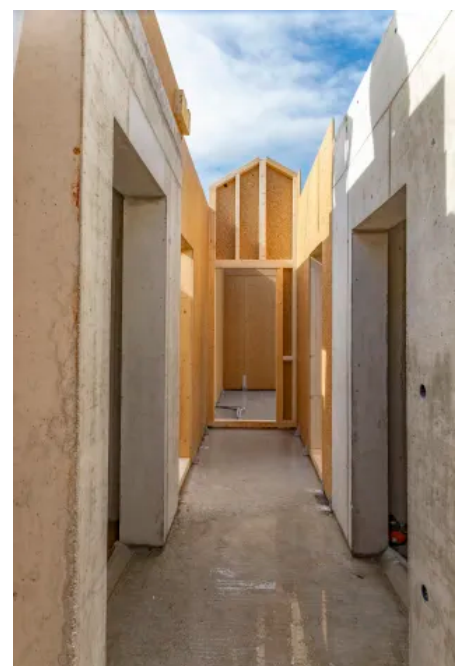
Hybridbauweise mit Holzrahmenbauelementen und Beton
