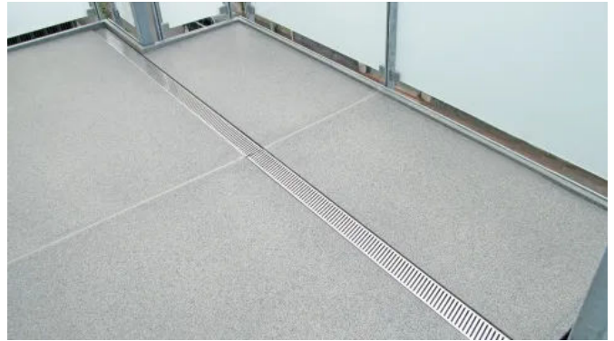
Detail Bakodur® E Holzzement-Gefälleplatten mit Ablaufrinne
