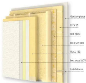
Wärmedämmverbundsystem mit best wood WALL 180 und best wood FLEX 50
