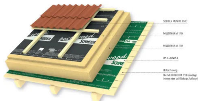
Aufdachdämmung mit best wood MULTITHERM 140 und 110
