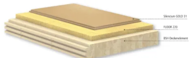
Bodendämmung mit best wood FLOOR 220
