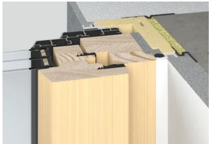
Premium-Montagesystem: Innen mit Verfugung
