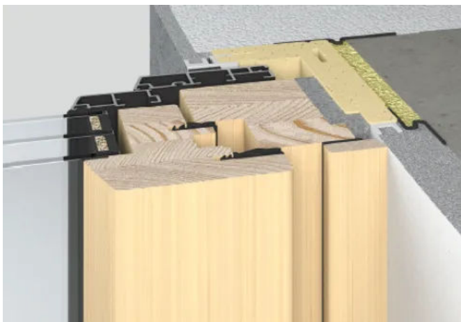
Premium-Montagesystem: Innen mit Standard-Deckelstreife
