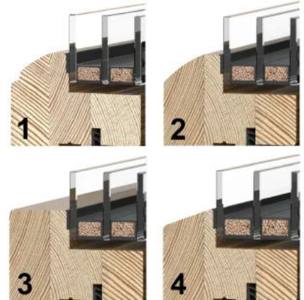
Innenprofilvarianten
