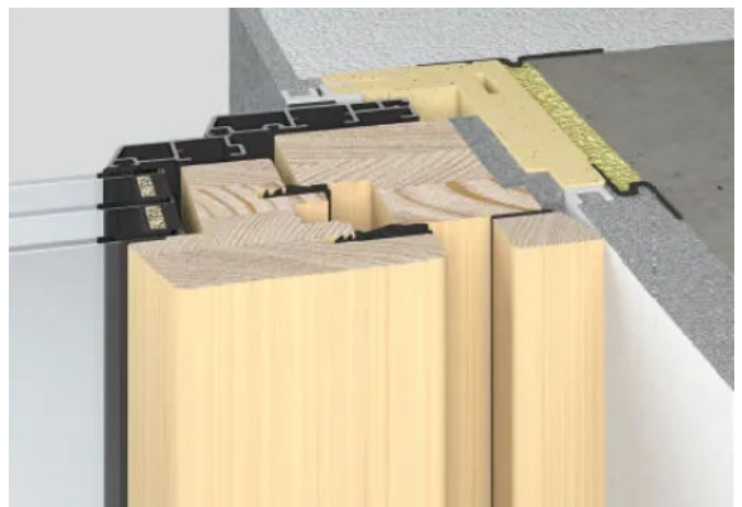
Premium-Montagesystem: Innen mit flächenbündiger Deckelstreife
