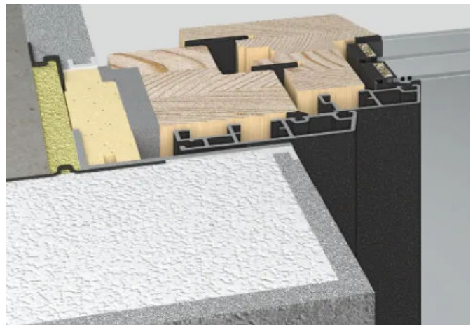
Premium-Montagesystem: Außen ohne Wärmedämmung
