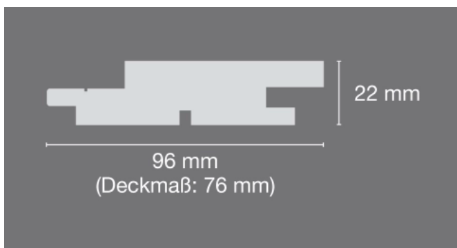
Deckmaß 76 mm
