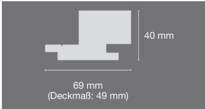
Deckmaß 49 mm
