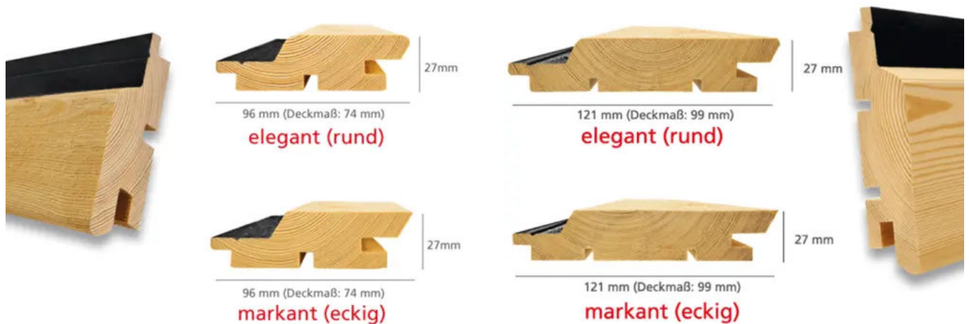
Trendliner Kontrast® - 96 mm
