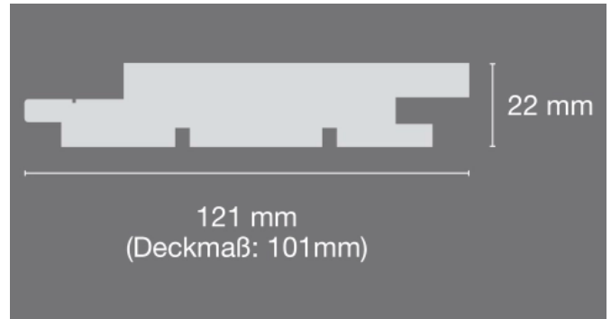
Deckmaß 101 mm
