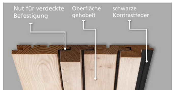
SKYLINE Kontrast - Befeuchtung
