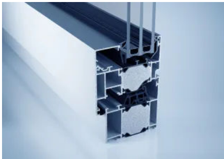
Fenstersystem heroal W 72 (© heroal)
