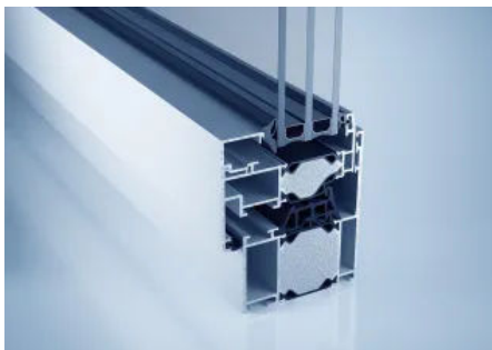
Fenstersystem heroal W 72 i (© heroal)
