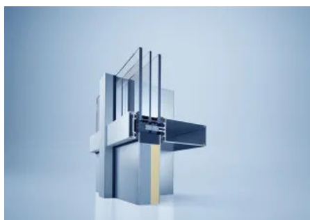
Fassadensystem heroal C 50 HI (© heroal)
