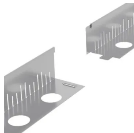
MONSUN® GREEN Dachrandprofil mit angeformten Stoßverbindern
