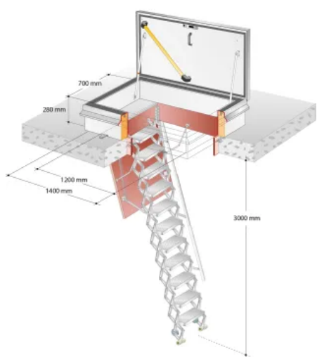
Sichere Dachausstiegslösung mit Scherentreppe (Typ Large). Auch eine optionale Verlängerung der Scherentreppe ist möglich.
