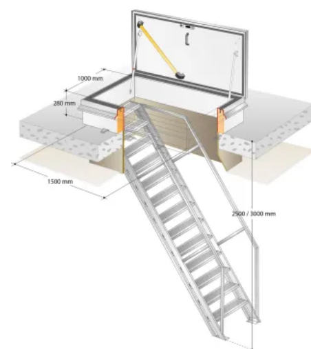
Der große Dachausstieg ergibt in Verbindung mit einer bauseits gefertigten Geschosstreppe eine komfortable Ausstiegslösung, sicherheitsgeprüft und wartungsarm!
