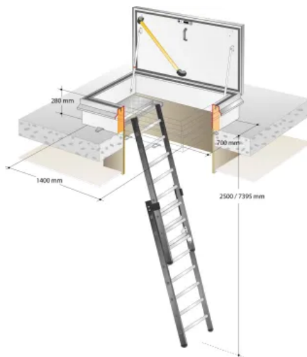
Alle Größen können mit einer fest angebauten Leiter kombiniert werden.
