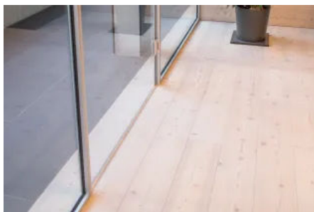
Gleiche Bautiefe von Glastür und Festfeldrahmen
