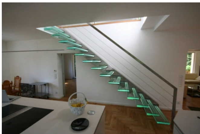
Leuchtglastreppe mit Wange (Kastenträger)
