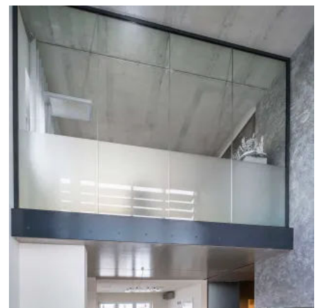
Galeriebüro: Absturzsicherung mit maßgefertigter Stahlkonstruktion.
