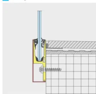
7 Anbindung seitlich an Balkon
