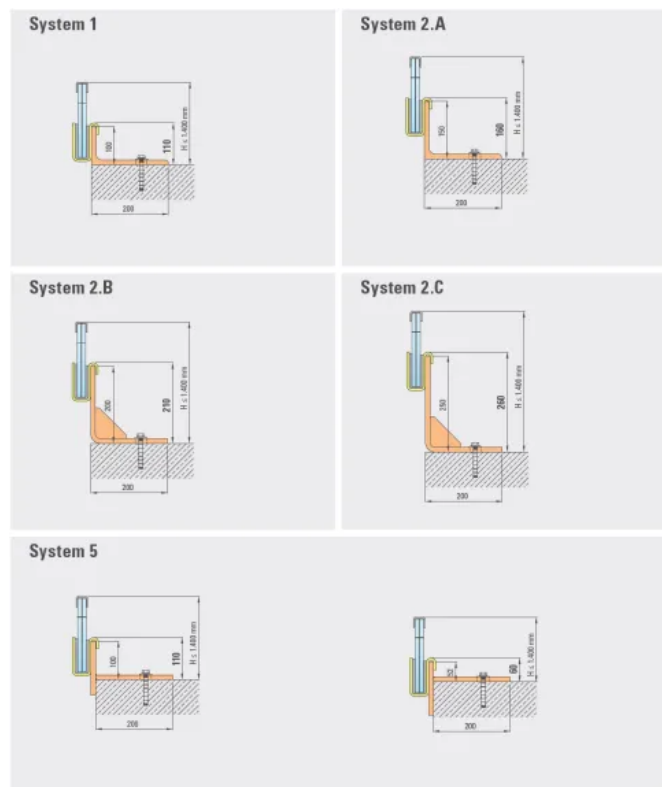
Anbindung an die Unterkonstruktion von oben bis 260 mm
