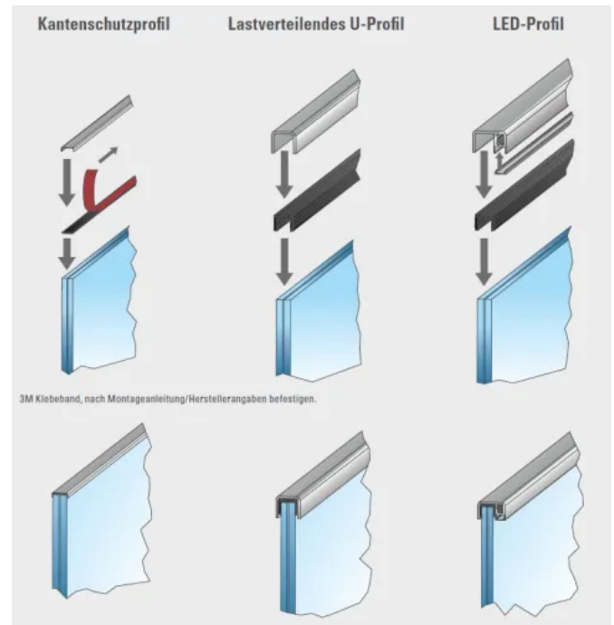
Montage Glaskantenschutzprofil und lastverteilende Handläufe
