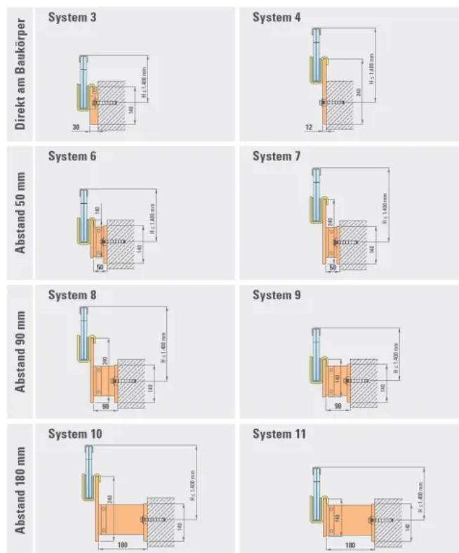
Anbindung an die Unterkonstruktion seitlich Abstand bis 180 mm
