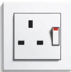
British Standard mit Shutter (Abbildung mit Gira E2)
