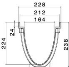
WOLFA MAXI Kastenrinnen Typ 150V
