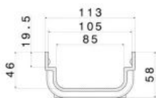
WOLFA-Flachrinne Typ 100/6
