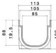
WOLFA-Kastenrinne Typ 100/8,5S
