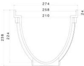
WOLFA MAXI Kastenrinnen Typ 200V
