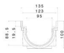
WOLFA-Kastenrinne Typ 100/8V
