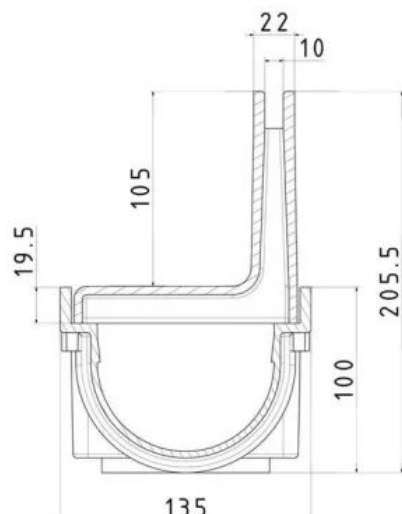
WOLFA-Schlitzrinne Typ 100/8VS-10,5
