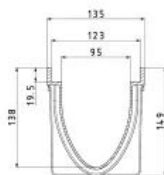
WOLFA-Kastenrinne Typ 100/V-Line
