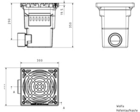
WOLFA Hofeinfüllkasten, Abmessungen
