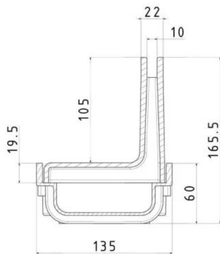
WOLFA-Schlitzrinne Typ 100/6VS-10,5
