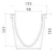
WOLFA-Kastenrinne Typ 100/10T
