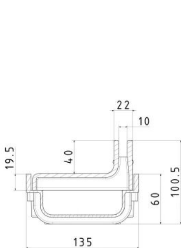
WOLFA-Schlitzrinne Typ 100/6VS-4
