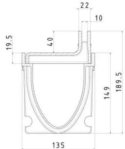
WOLFA-Schlitzrinne Typ 100VS-4
