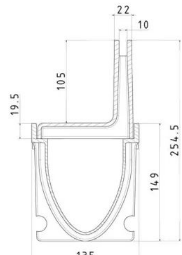
WOLFA-Schlitzrinne Typ 100VS-10,5
