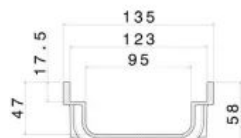
WOLFA-Flachrinne Typ 100/6V
