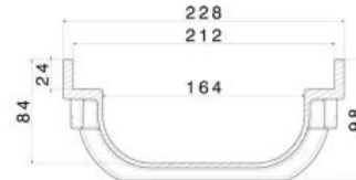
WOLFA-Flachrinne Typ 150F
