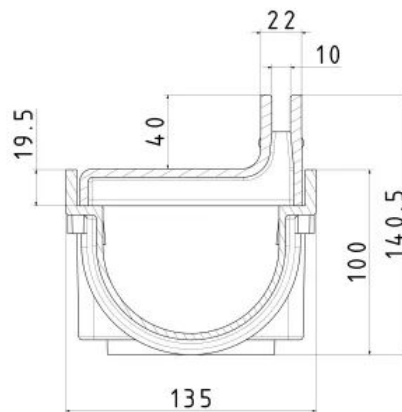
WOLFA-Schlitzrinne Typ 100/8VS-4
