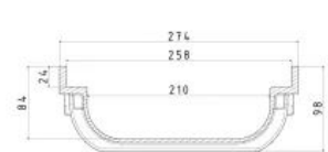
WOLFA-Flachrinne Typ 200F
