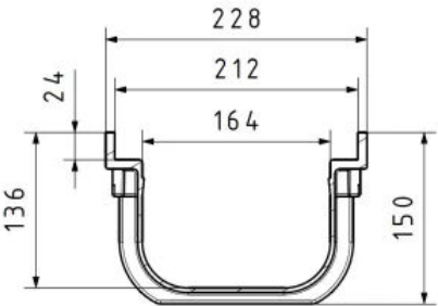
WOLFA-Kastenrinne Typ 150K
