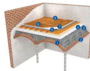
Systemskizze: Gewölbedämmung mit GEOMATERIALS Blähglas
