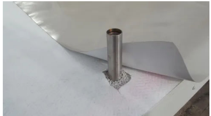
Optimale Einbindung von Abflüssen und Rohrdurchführungen ohne zu schneiden
