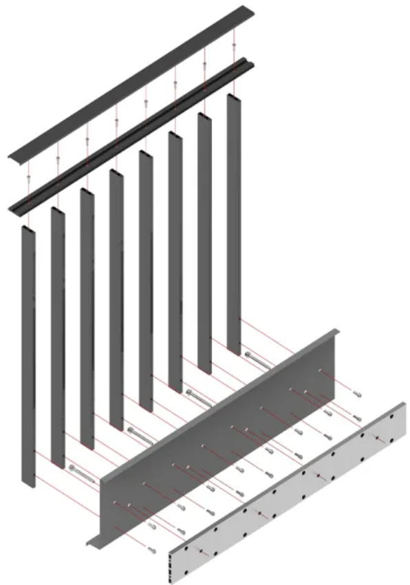
Schematischer Aufbau Stabgeländer LAMINA
