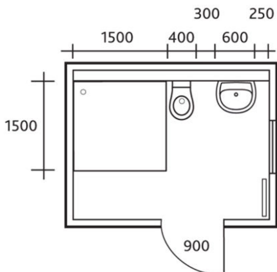
Umbau Bad mit größerem Duschplatz für Rollstuhlbenutzer
