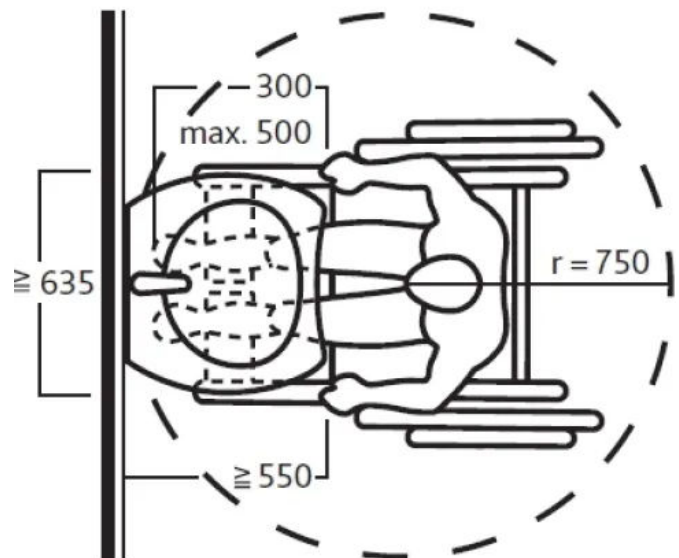
Maßangaben in mm, Zeichnung in Anlehnung an Sanitär-Technik, Feurich/Kühl, Band 1, 2011
