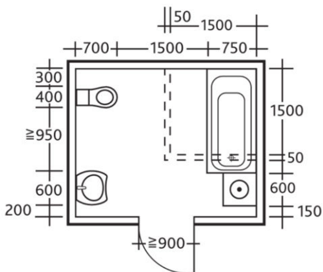
Grundriss-Beispiel Baderaum für Rollstuhlbenutzer
