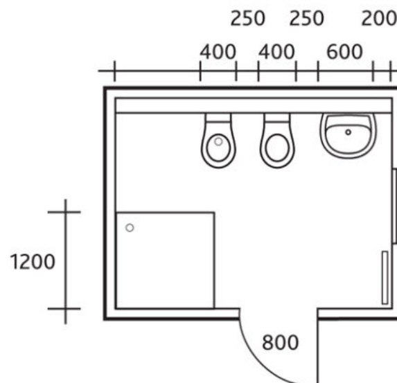
Umbau Bad mit größerer, bodengleicher Duschwanne
