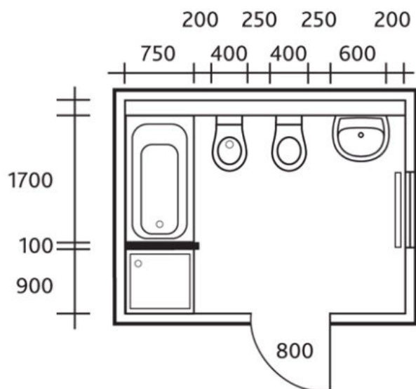
Bad mit Dusche und Badewanne (Ausgangssituation)
