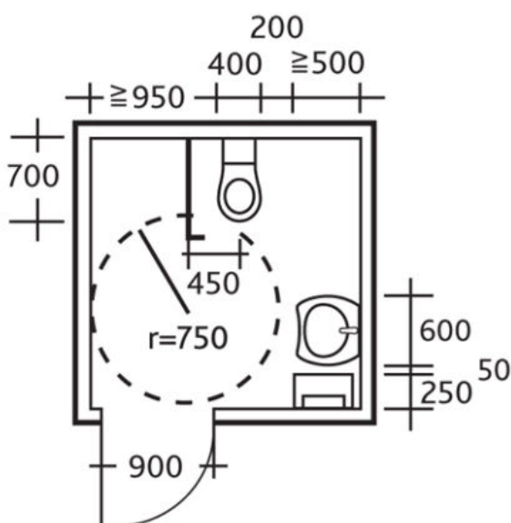
Grundriss-Beispiel WC-Raum für Rollstuhlbenutzer
