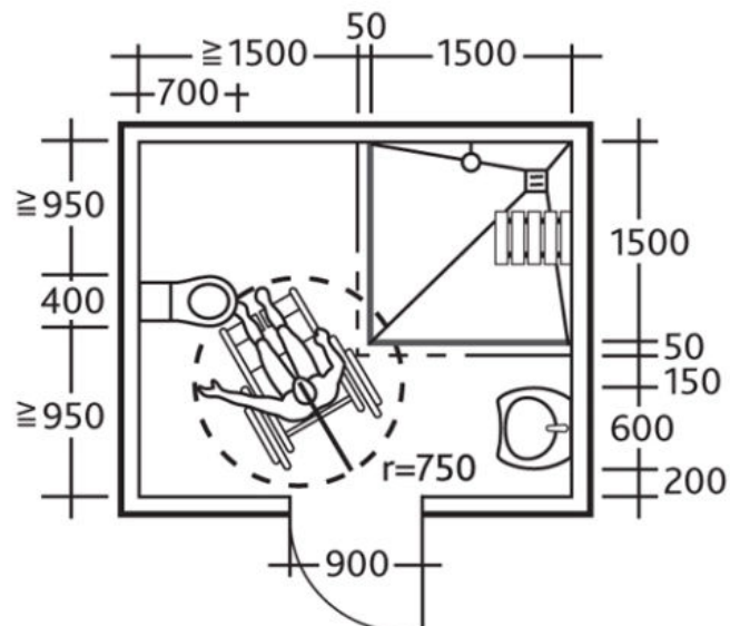
Grundriss-Beispiel für rollstuhlgerechte, barrierefreie Duschbäder
