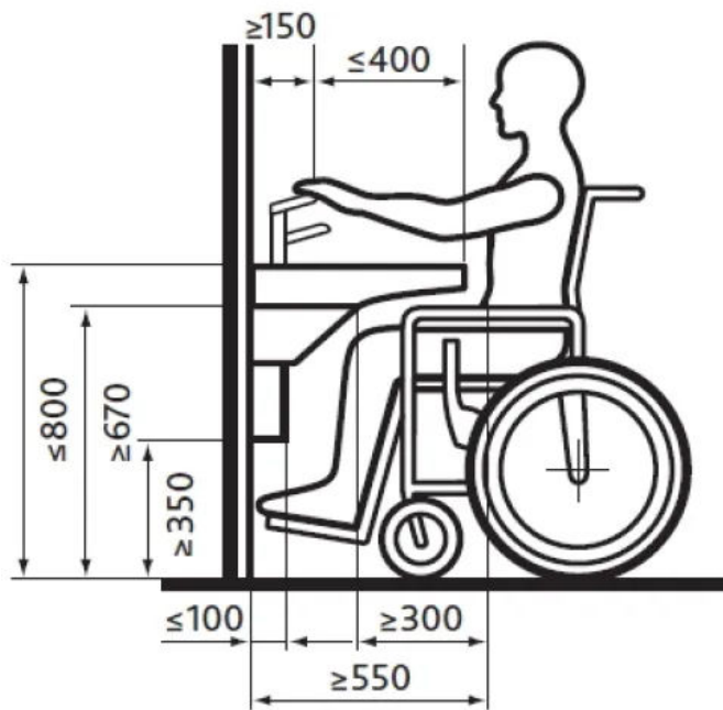
Maßangaben in mm, Zeichnung in Anlehnung an DIN 18040-1 Barrierefreies Bauen (10/2010)
