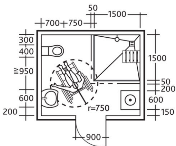
Grundriss-Beispiel für rollstuhlgerechte, barrierefreie Duschbäder
