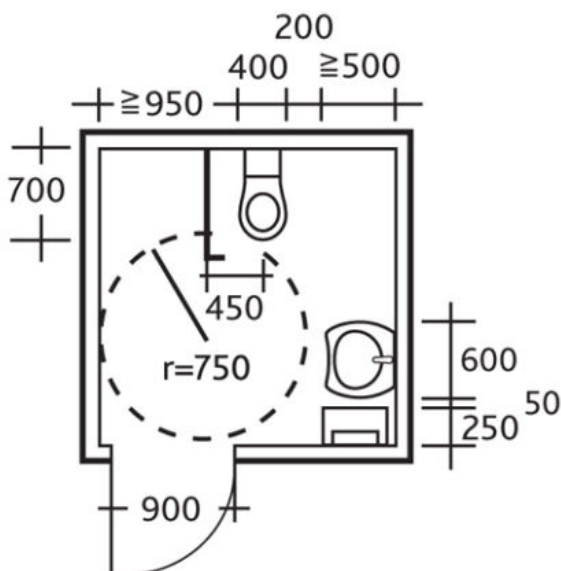
Grundriss-Beispiel WC-Raum für Rollstuhlbenutzer
