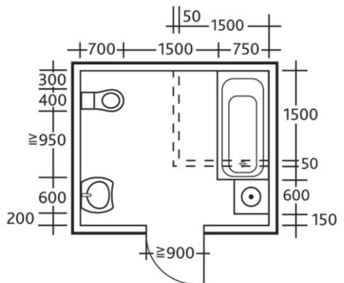
Grundriss-Beispiel Baderaum für Rollstuhlbenutzer
