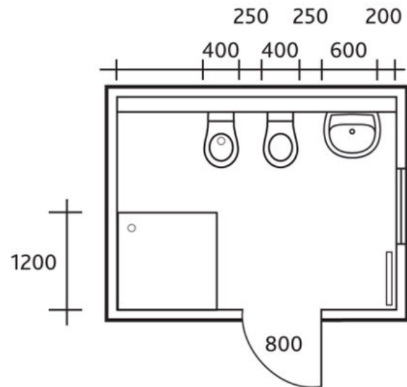
Umbau Bad mit größerer, bodengleicher Duschwanne
