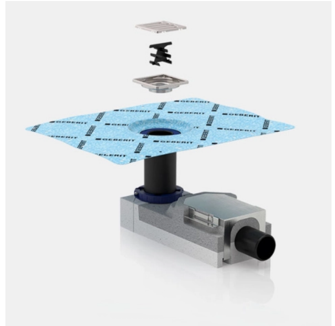
Der Grundkörper des CleanPoint Bodenablaufs ist mit einem flexiblen Abdichtvlies ausgestattet.
