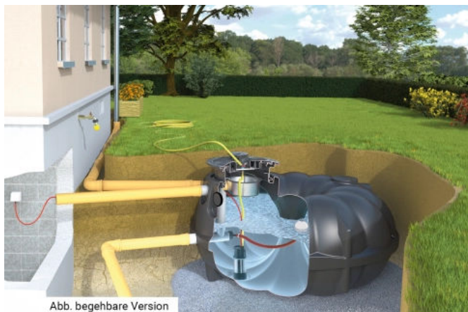
Garten-Komplettanlage Retention und Nutzung – Regenwassernutzung kombiniert mit Rückhaltung mit Wasseranschluss im Tankdeckel
