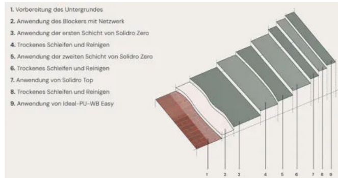
Solidro - Systemaufbau 2, für Wand, Boden und auch bestehenden Bodenbelägen wie Keramikfliesen oder Naturstein.
