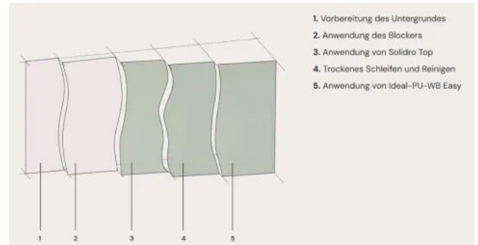
Solidro - Systemaufbau 3, für einfache Wände
