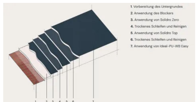
Solidro – Systemaufbau 1-Standard, Wand und Boden
