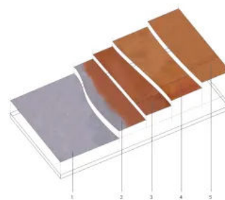
Acid Stain Dekorboden – Systemaufbau
