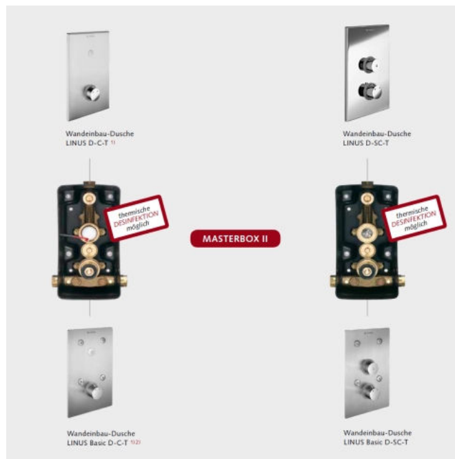
Masterbox II mit eingebauter Thermostatarmatur
