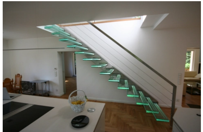
Leuchtglastreppe mit Wange (Kastenträger)
