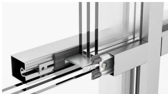
Hochwärmedämmte Vorhangfassade forster thermfix vario Hi
