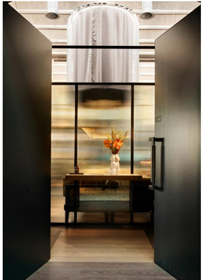
forster fuego light Flächenbündige Blechtür EI30, Foto: Bild: Beat Brechbühl
