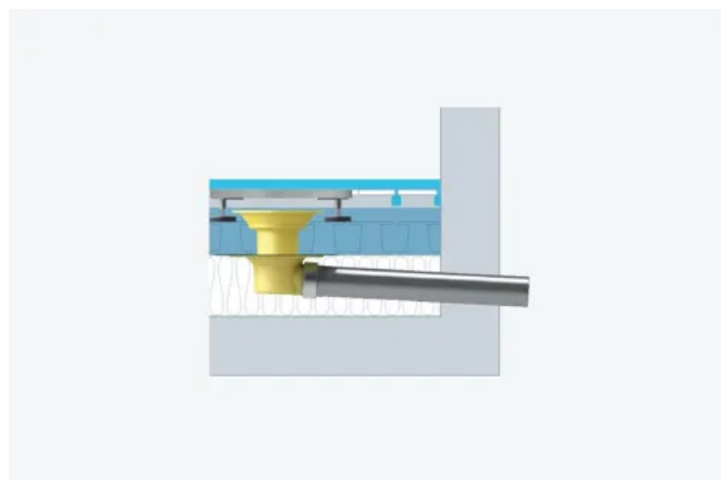
B. Als Speier eingesetzt: Sita Compact, abgewinkelt
