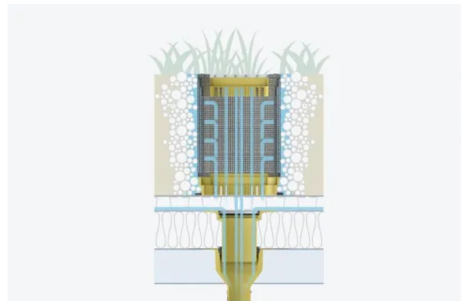
Für extensive und intensive Dachbegrünung: SitaGreen Gründachschacht
