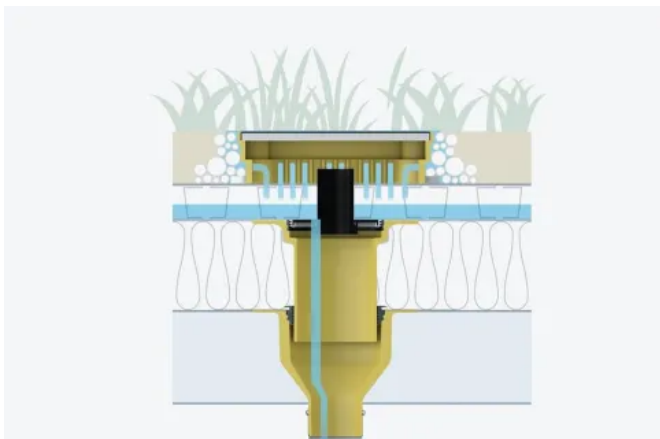
Zur verzögerten Entwässerung: SitaRetention Fix
