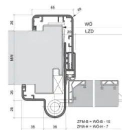
Modell RENOFI als Renovierungs-Umfassungscharge für die Kombination mit Küffner Fingerschutztür
