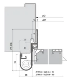
Modell EFI als Renovierungs-Eckzarge für die kostengünstige Sanierung und geringster Reduzierung des lichten Durchgangs
