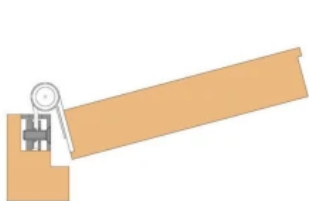
Das Schutzprofil BD reduziert die Stoßgefahr direkt am Band.
