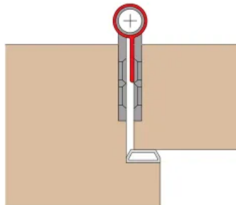
Schutzprofile B0-13 und B0-23 für stumpfe Holztüren
