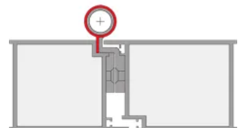
Schutzprofile B0-20 und B0-22 für flächenbündige Profiltüren
