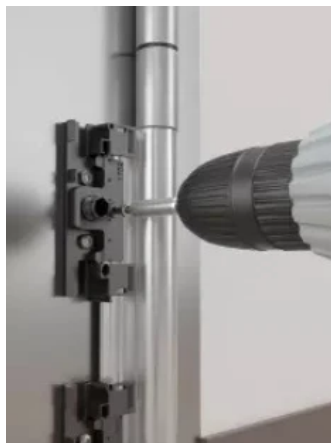
Anschrauben mit passenden Bohrschrauben ohne Vorbohren und Senken
