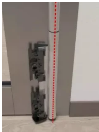
Ausrichten in der Flucht des Bandes und Andrücken der Profile mit Klebepads
