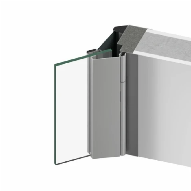
Bandseitiges Schutzprofil BSG1
