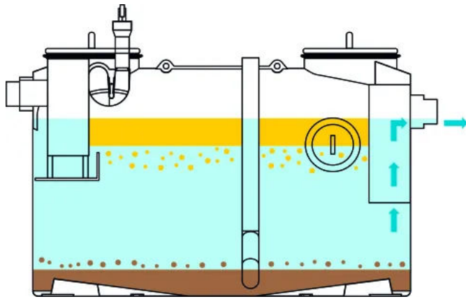
4. Ableiten des gereinigten Wassers
