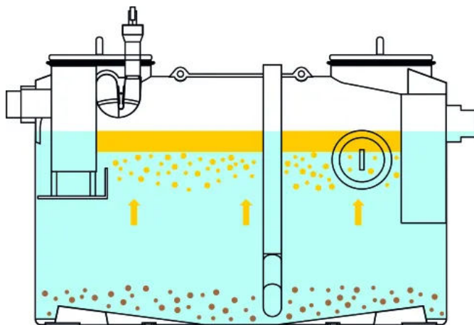
3. Aufsteigen von Fetten und Ölen
