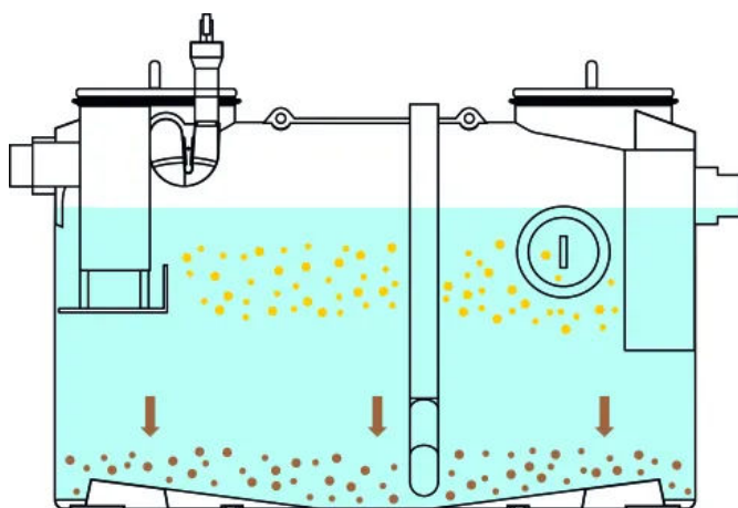
2. Absetzen schwerer Stoffe im Schlammfang
