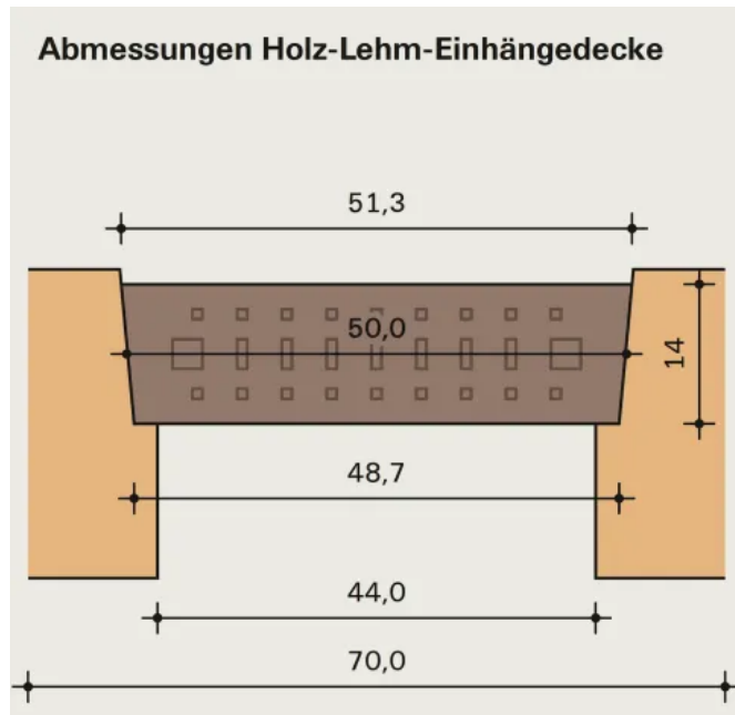
Maße Holz-Lehm-Einhängedecke
