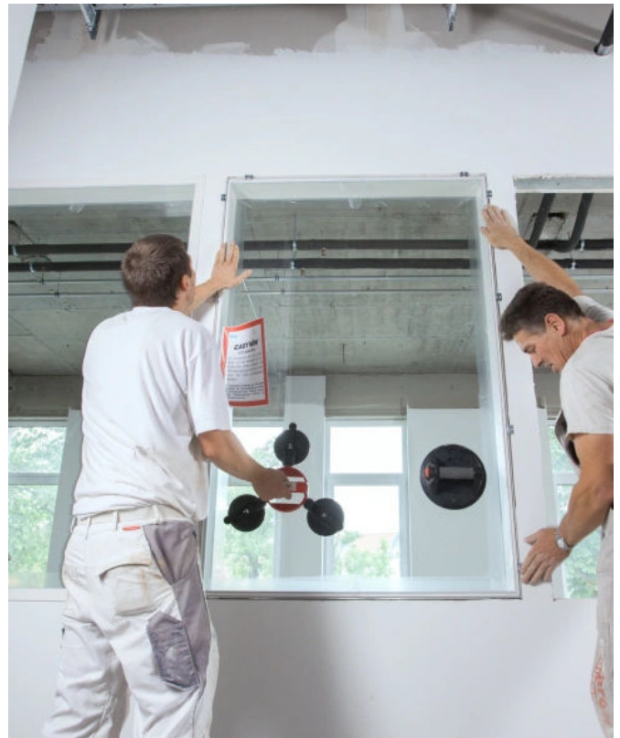
Die EasyWin Fertigfenster werden montagefertig als Monoblock mit wandbündiger Doppelverglasung auf die Baustelle geliefert.
