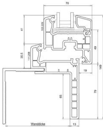
Profilquerschnitt Klickfix 70, hier Kipflügeleinsatz Typ TOP
