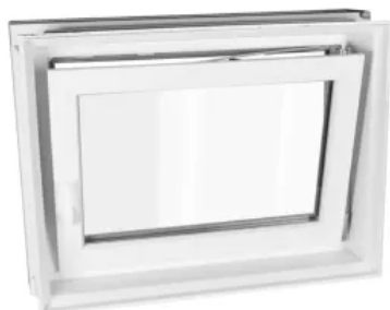
Zargenfenster Typ Z 82 wärmegeklämt, komplett mit Drehkipplügel
