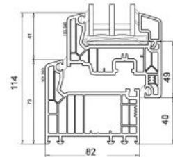
Profilquerschnitt 7-Kammerprofil Typ MDK de Luxe 82 mit bester Wärmedämmung ( U_w 0,85 \text{ W/m}^2\text{K} )
