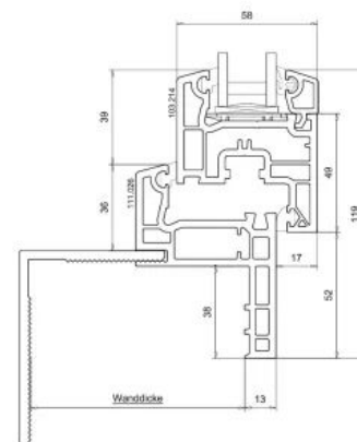
Profilquerschnitt Klickfix 58, hier Kipflügeleinsatz Typ TOP
