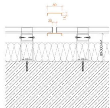
S03 PRO+ Querstoß
