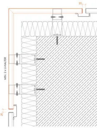
S02 PRO+ Eckausbildung
