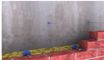
MOSO® HV-D Drahtanker für die nachträgliche Horizontalverbindung
