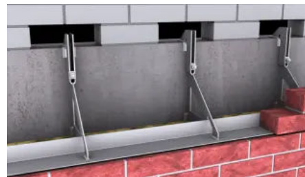
MOSO® Winkelkonsolanker WK-K für niedrige Betonhöhen
