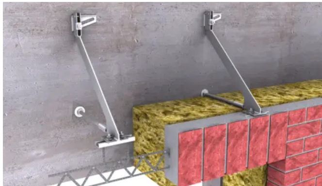
MOSO® Fertigteilbefestigung FB-D mit justierbarer Druckschraube
