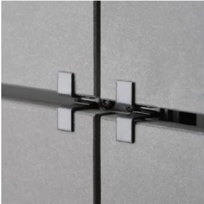
Detailansicht – sichtbares Doppelklammersystem zur mechanischen Befestigung keramischer Mosa-Fassadenplatten.
