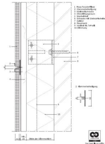
Vertikalschnitt – konstruktiver Aufbau der hinterlüfteten Fassade mit sichtbarer Doppelklammerbefestigung auf Aluminium-Unterkonstruktion.
