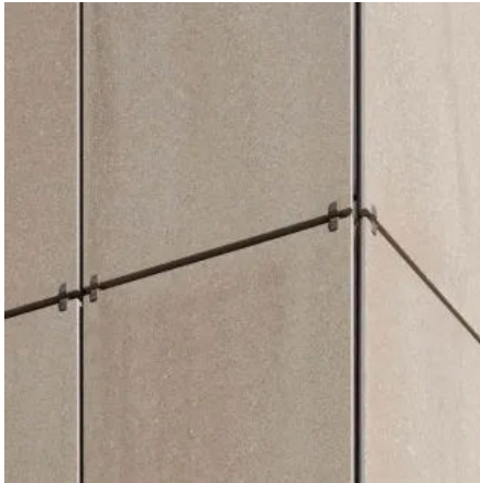
Facettenecken – nahtlose Eckausbildung für ein harmonisches Fassadenbild.
