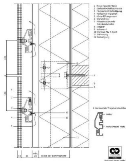
Vertikalschnitt – konstruktiver Aufbau einer hinterlüfteten Fassade mit unsichtbarer Befestigung und Aluminium-Unterkonstruktion.
