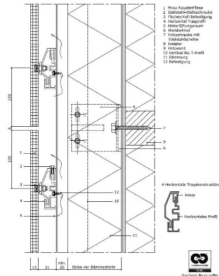
Vertikalschnitt
