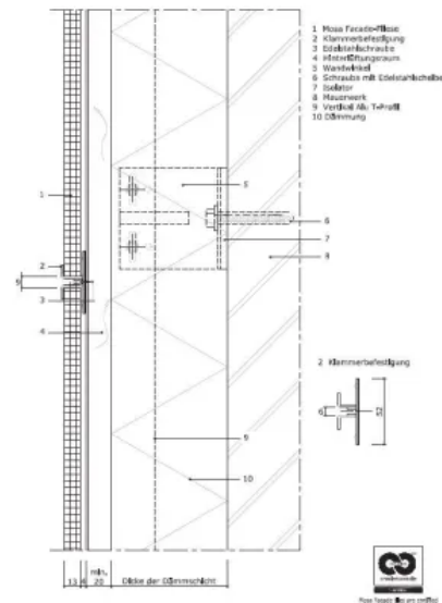
Vertikalschnitt
