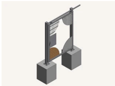
Hängeschiebetor einflügelig
