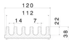
AquaStop Klassik, 120 x 38 mm
