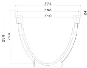
WOLFA MAXI Kastenrinnen Typ 200V
