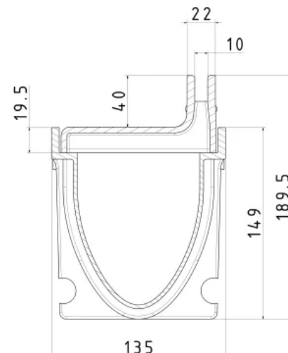
WOLFA-Schlitzrinne Typ 100VS-4
