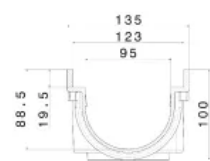
WOLFA-Kastenrinne Typ 100/8V
