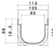
WOLFA-Kastenrinne Typ 100/8,5S
