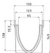
WOLFA-Kastenrinne Typ 100/V-Line
