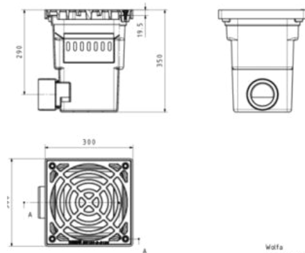
WOLFA Hofeinführungskasten, Abmessungen
