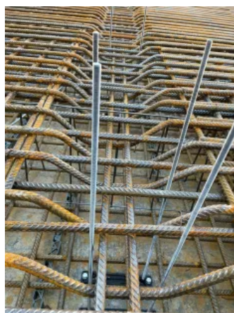
Bewehrung einbauen und Gewindestangen montieren.
