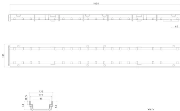
WOLFA Reihe 100/6V Drain
