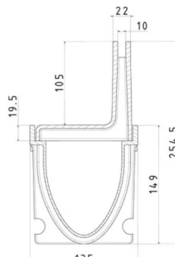
WOLFA-Schlitzrinne Typ 100VS-10,5
