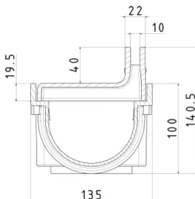
WOLFA-Schlitzrinne Typ 100/8VS-4
