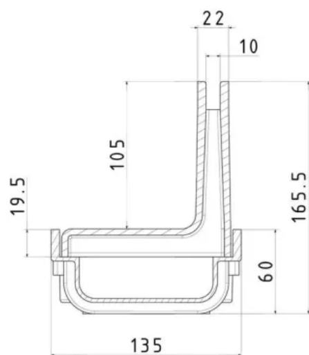
WOLFA-Schlitzrinne Typ 100/6VS-10,5
